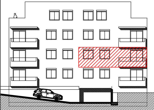
ISTOČNO PROČELJE
