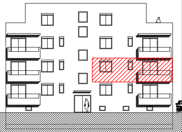
ZAPADNO PROČELJE
