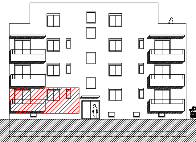
ZAPADNO PROČELJE
