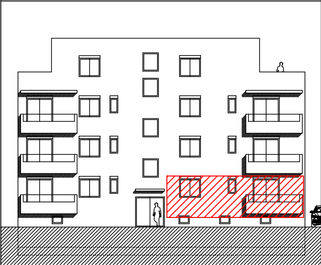
ZAPADNO PROČELJE
