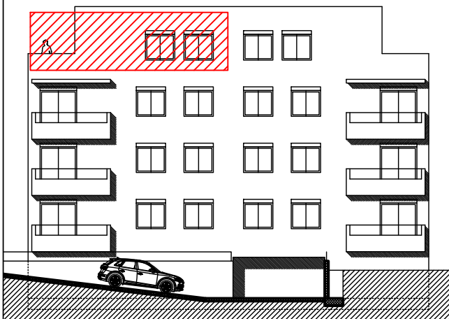
ISTOČNO PROČELJE
