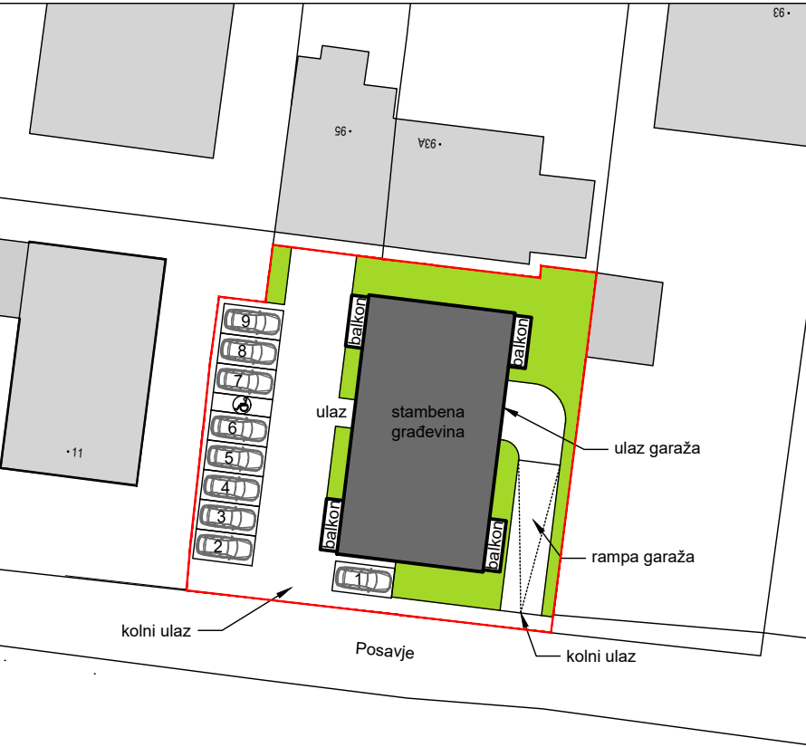
SITUACIJA
